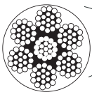
Cable flexible 7 x 19 hilos
