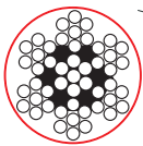
Cable rígido 7 x 7 hilos
